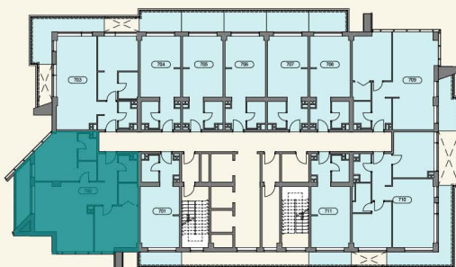
План этажа
