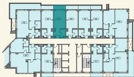
План этажа
