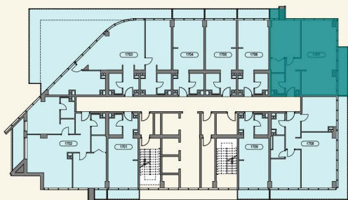
План этажа
