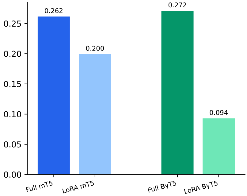
Token F1
