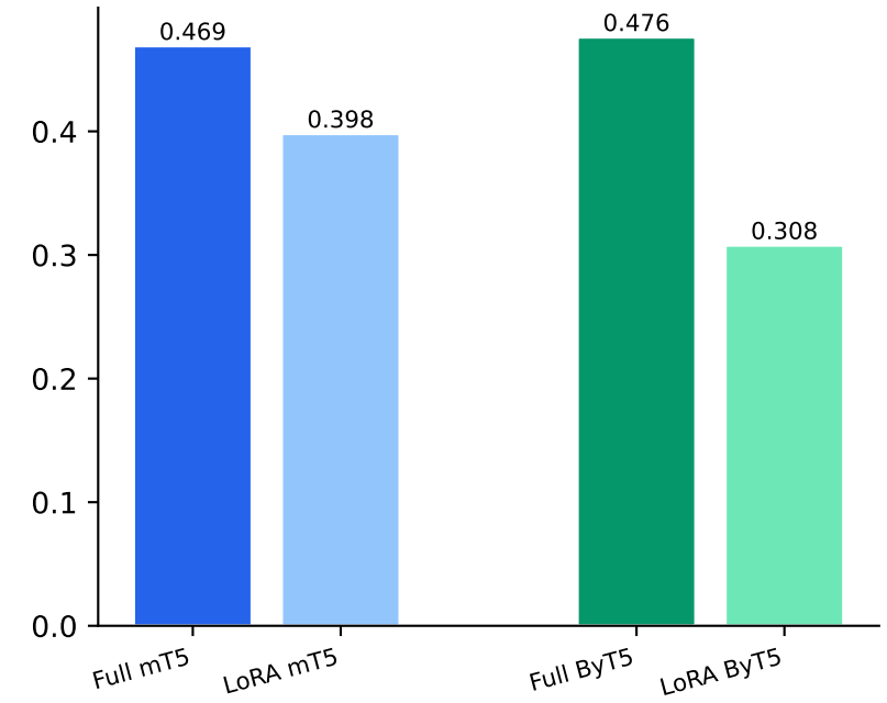
Semantic Sim.
