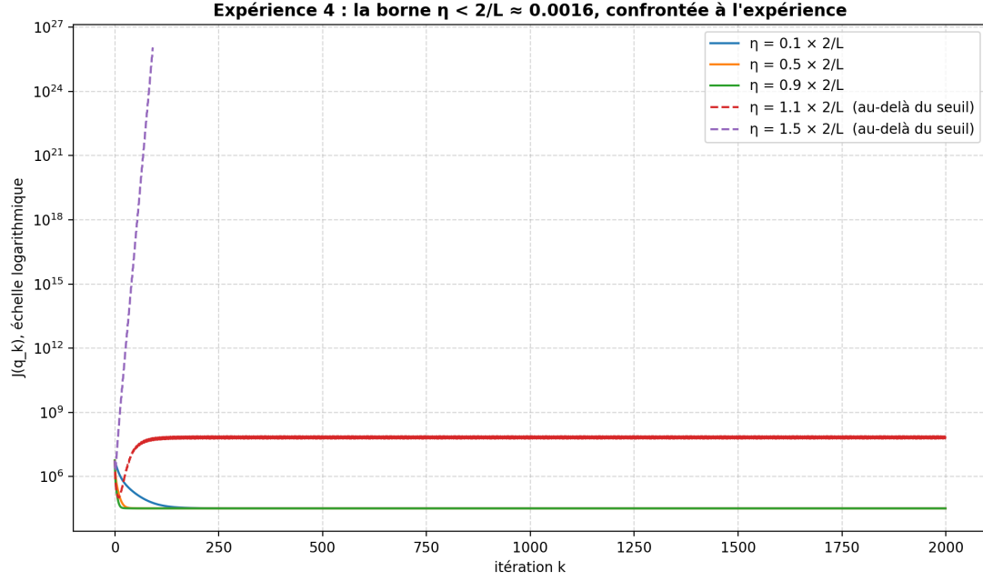
Figure 5: Confrontation expérimentale à la borne théorique \eta < 2/L .
