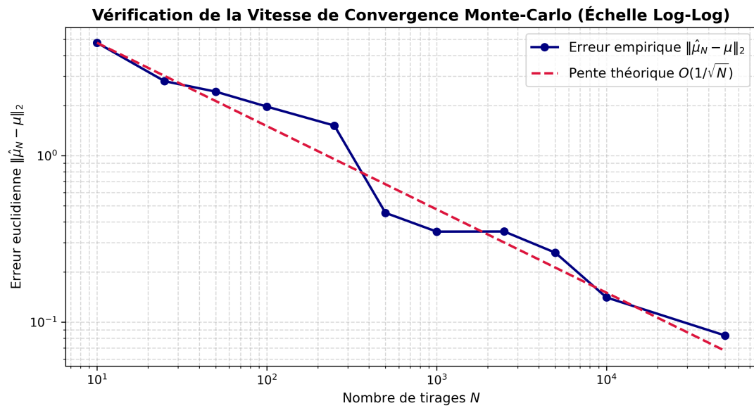
Figure 9: Convergence de la moyenne empirique et erreur d'estimation.
