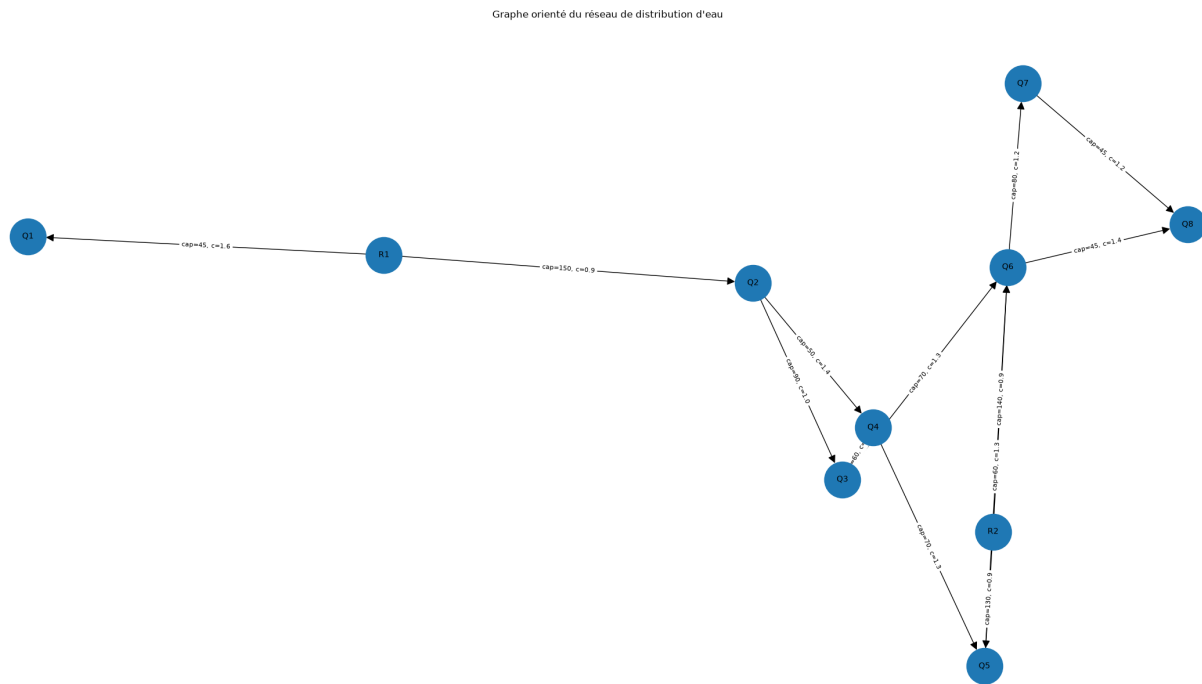
Figure 13: Représentation topologique orientée du réseau d'eau, illustrant les réservoirs \{R_1, R_2\} , les quartiers \{Q_1, \dots, Q_8\} , les arêtes-ponts vers Q_1 et la redondance maillée de la zone aval.
