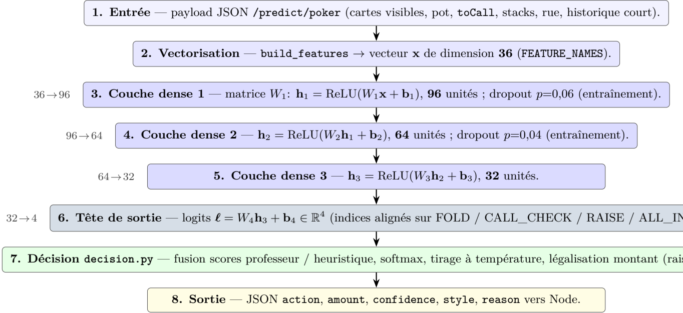
Figure 1: Flux de données du prototype MLP expert ( ExpertPolicy ): vecteur de 36 caractéristiques, couches denses, puis post-traitement métier avant réponse HTTP.
