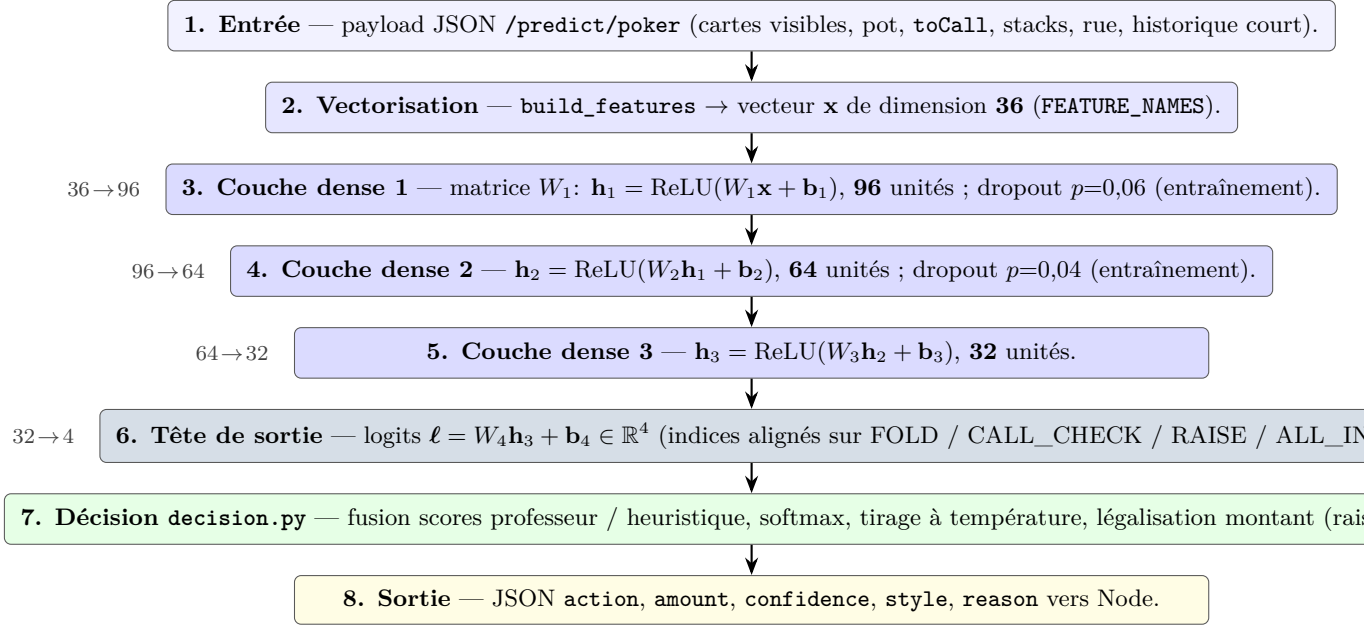
Figure 1: Flux de données à travers la politique MLP expert ( ExpertPolicy ): 4 transformations linéaires successives, 196 neurones après la couche d’entrée (96+64+32+4), puis post-traitement métier avant réponse HTTP.
