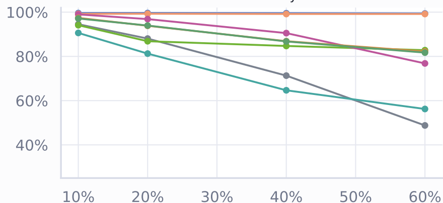
UNSW-NB15: symmetric
