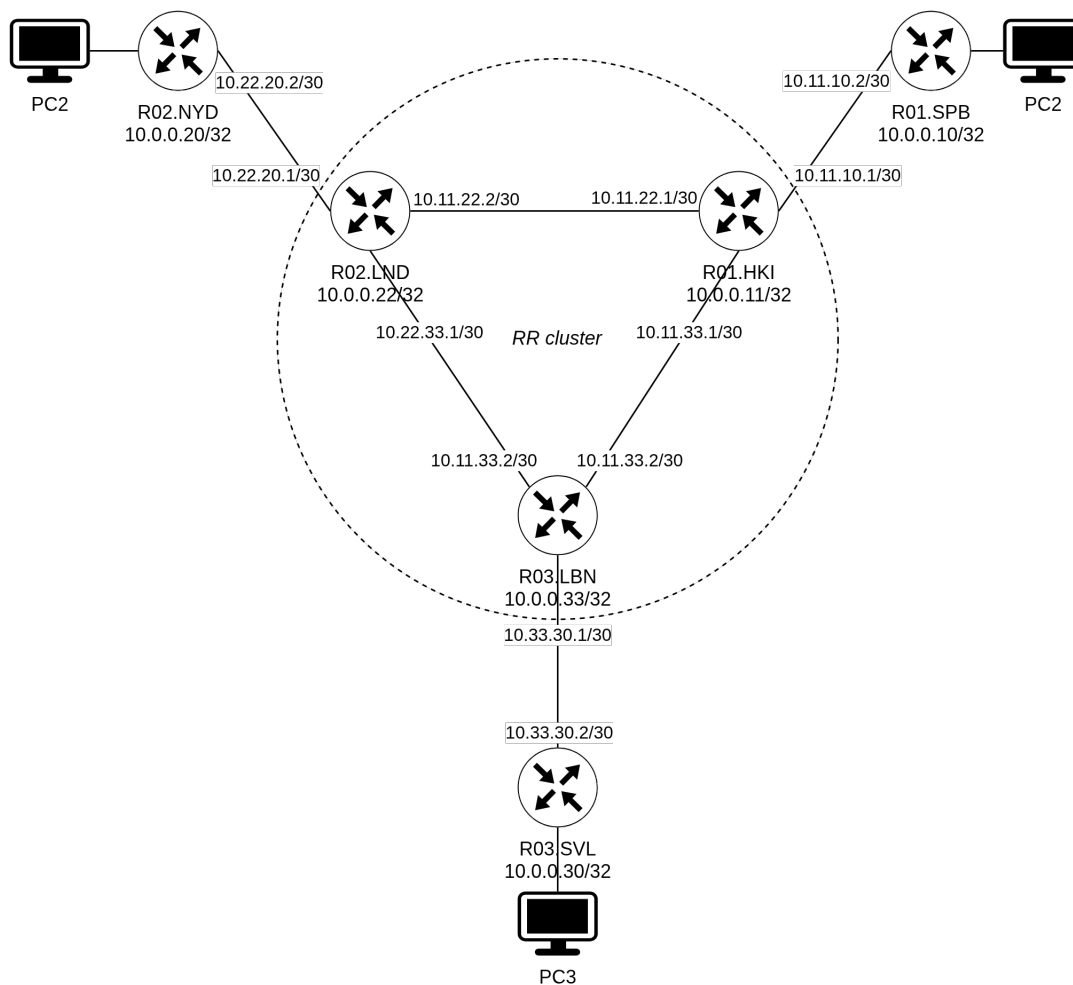
Рисунок 1.2 — Схема сети
