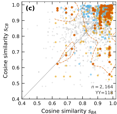
Type 3: A \leftarrow B \leftarrow C
