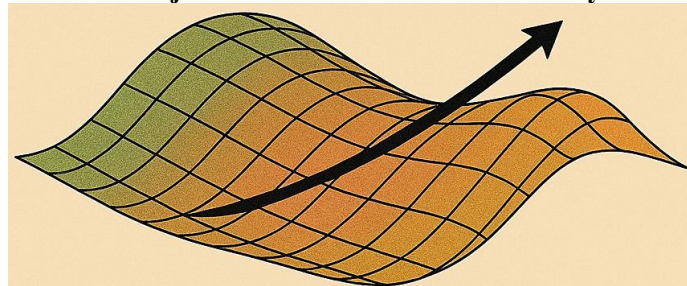
Figura 5. El Tao como flujo armónico modelado en una trayectoria geotensorial.
