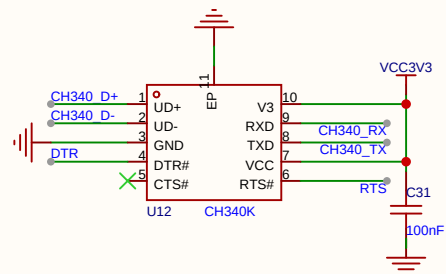
USB转UART
