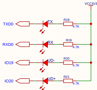
收发指示灯
