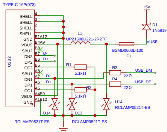
Type-C16
