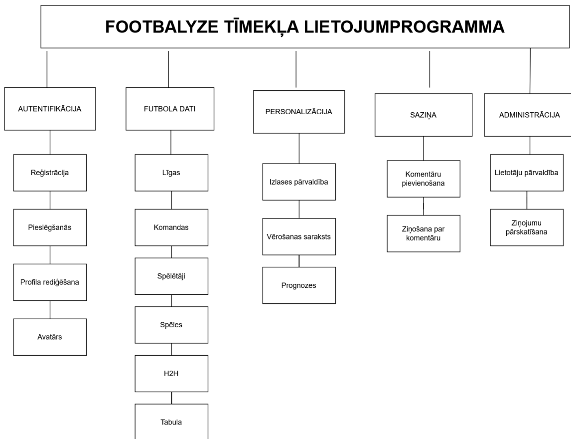
4.1.att.. Footbalyze funkcionālās dekompozīcijas diagramma
