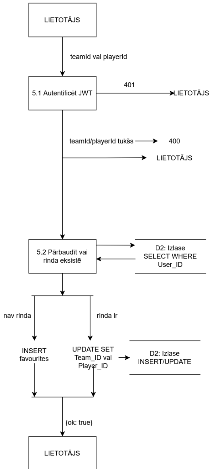
4.8.att.. Izlases pārvaldības moduļa datu plūsmas diagramma
