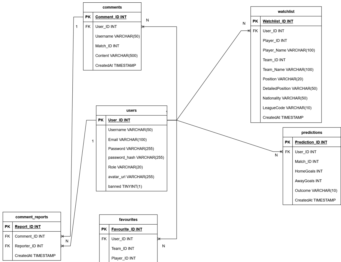
5.1.att.. Datubāzes tabulu saišu shēma
