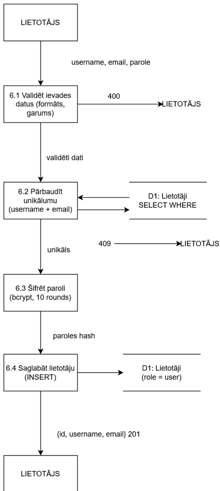
4.6.att.. Reģistrācijas moduļa datu plūsmas diagramma
