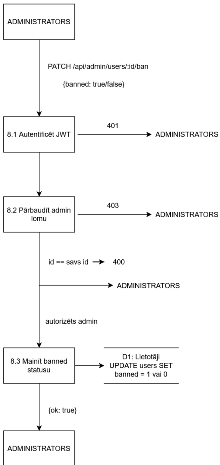
4.10.att.. Lietotāja bloķēšanas moduļa datu plūsmas diagramma
