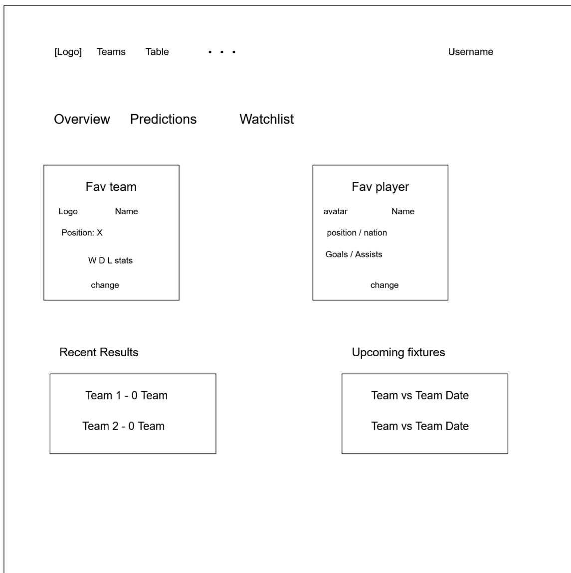
2.3.att.. Lietotāja paneļa ekrānloga skice
