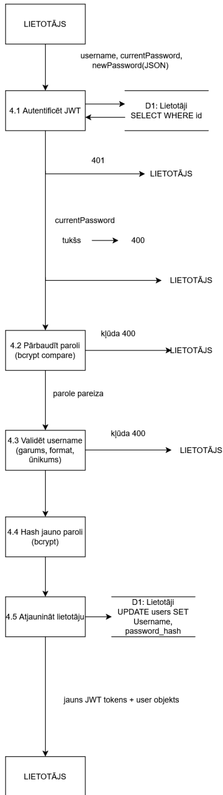
4.7.att.. Profila rediģēšanas moduļa datu plūsmas diagramma
