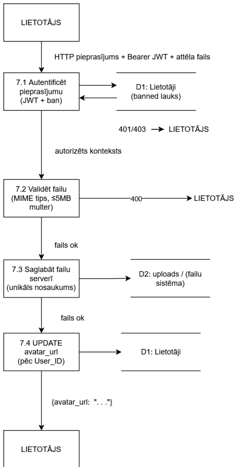
4.9.att.. Avatāra augšupielādes moduļa datu plūsmas diagramma
