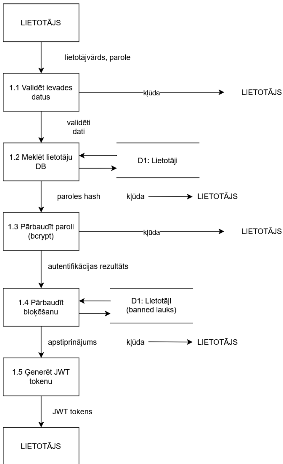
4.3.att.. Lietotāja pieslēgšanās moduļa datu plūsmas diagramma
