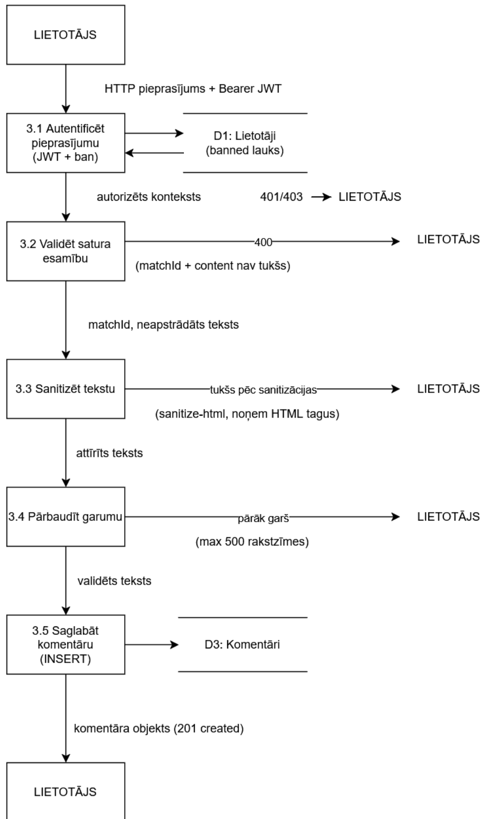
4.5.att.. Komentāra pievienošanas moduļa datu plūsmas diagramma
