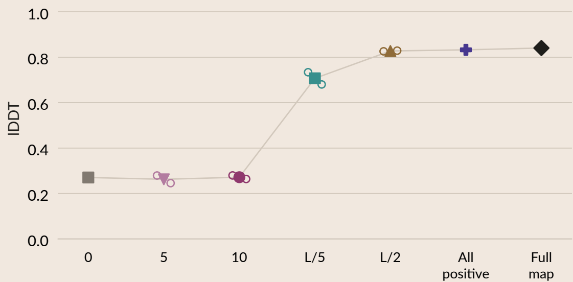
8qoh_A • depth 3 • L = 278
