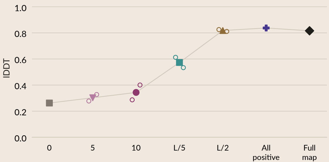
8ux2_A • depth 6 • L = 246
