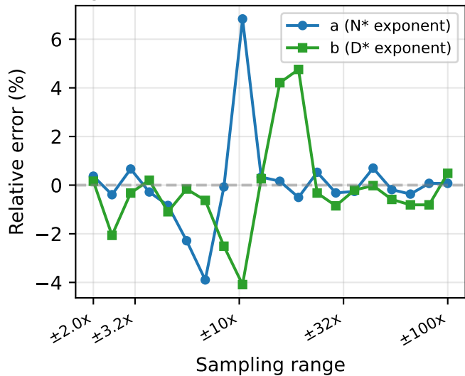
Exponent Error
