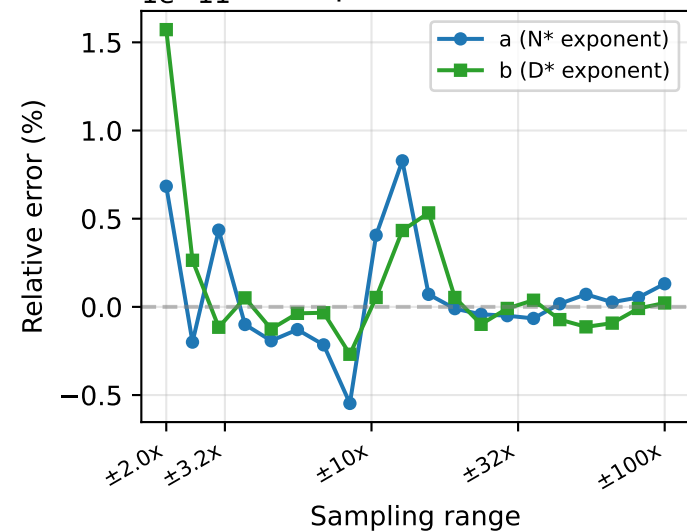
Exponent Error
