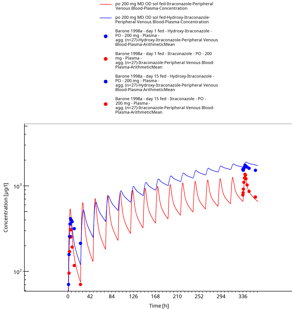
Figure 3-27: po 200 mg MD OD sol fed - Plasma
