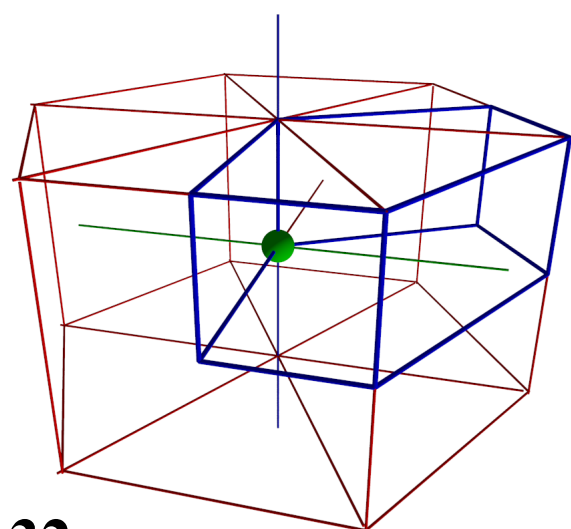
32
