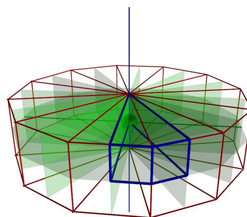
6/mmm
