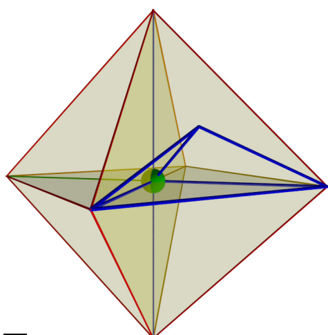
m\bar{3}
