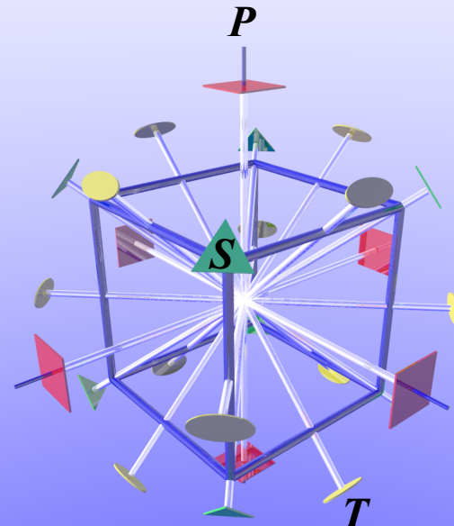
(f) Cubic
