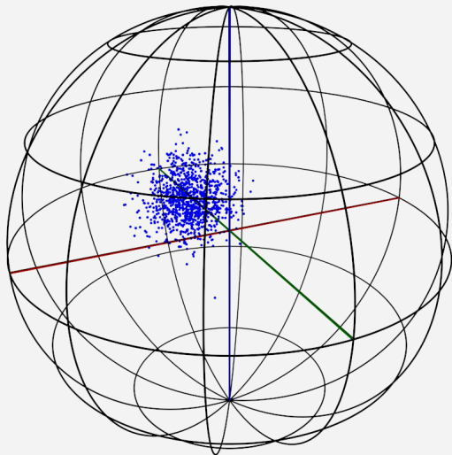
(a) von Mises-Fisher
