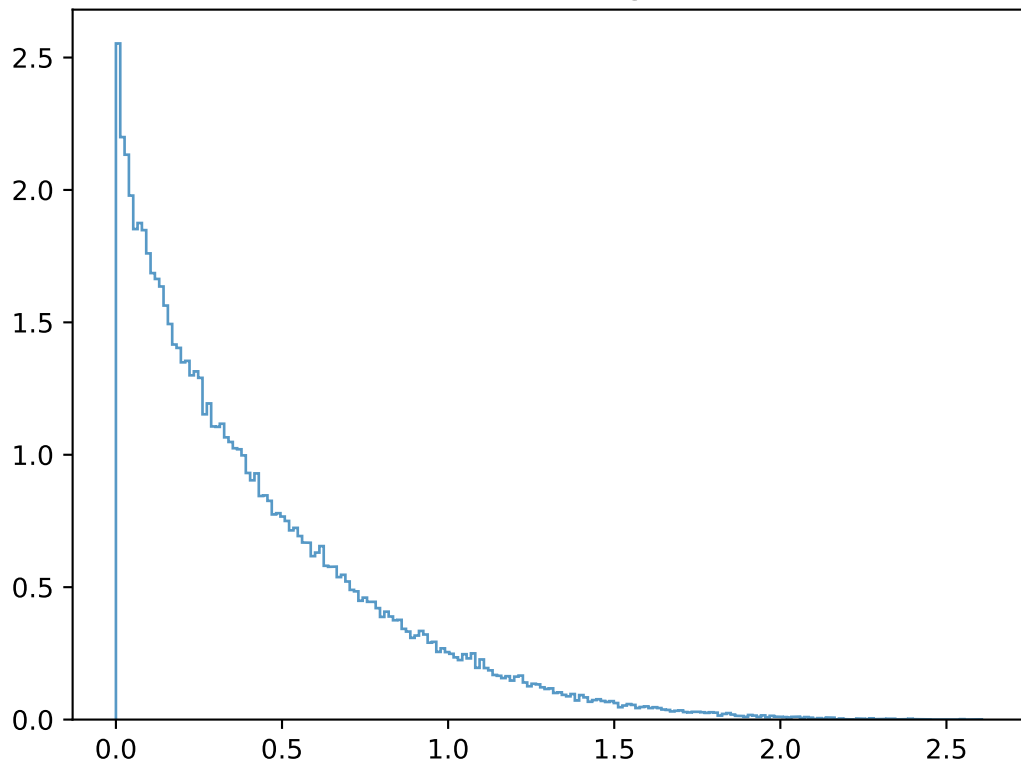
Positron range
