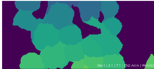
E Labels
