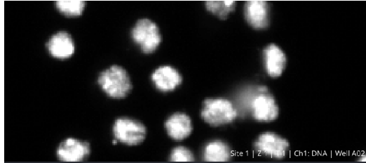
A Raw
