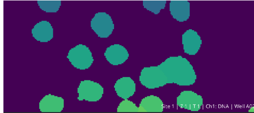
B Labels
