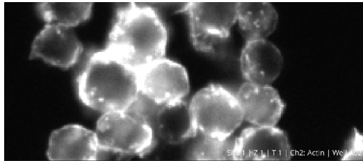
D Raw
