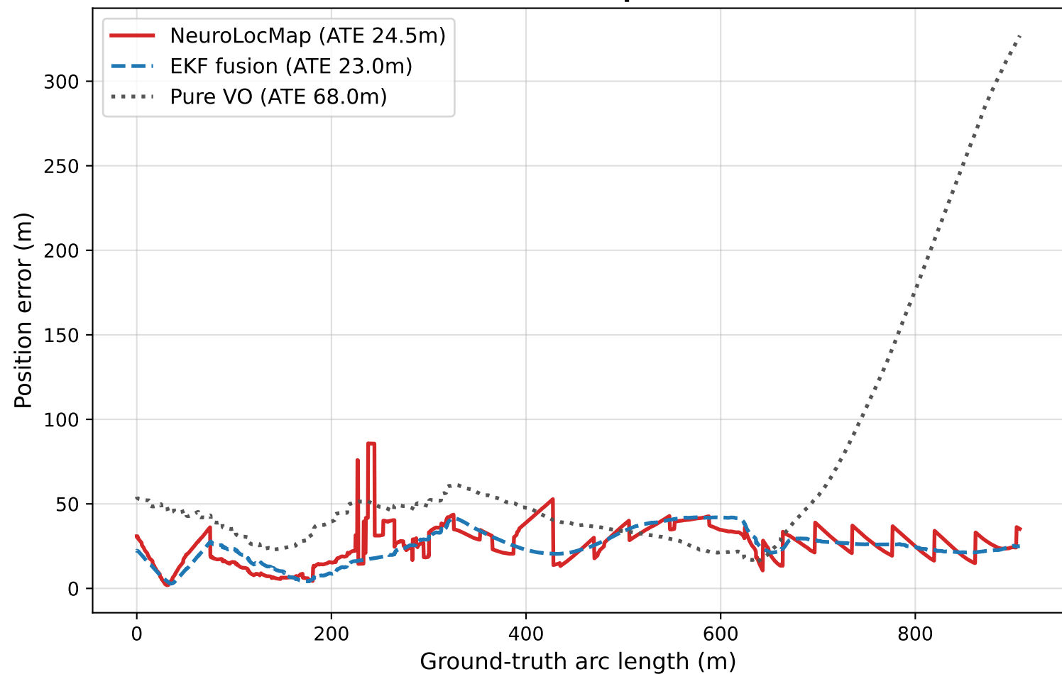
Town05 NeuroLocMap vs EKF vs VO
