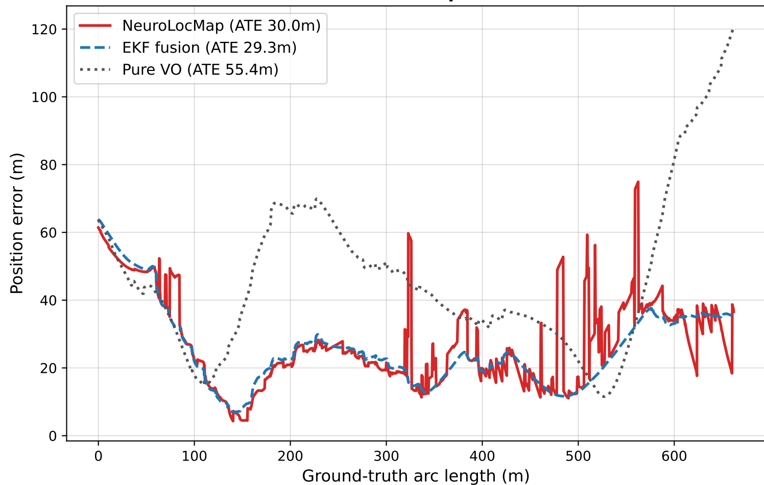
Town02 NeuroLocMap vs EKF vs VO
