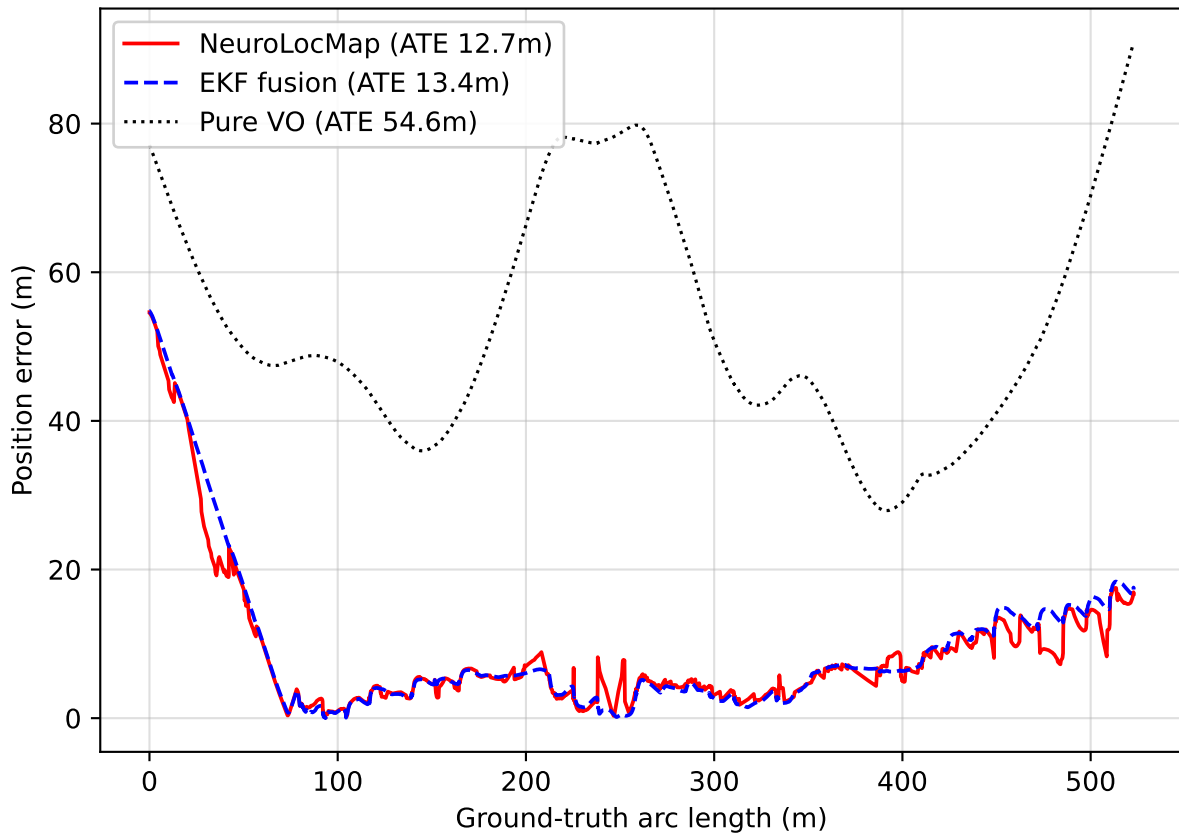
Town10HD NeuroLocMap vs EKF vs VO
