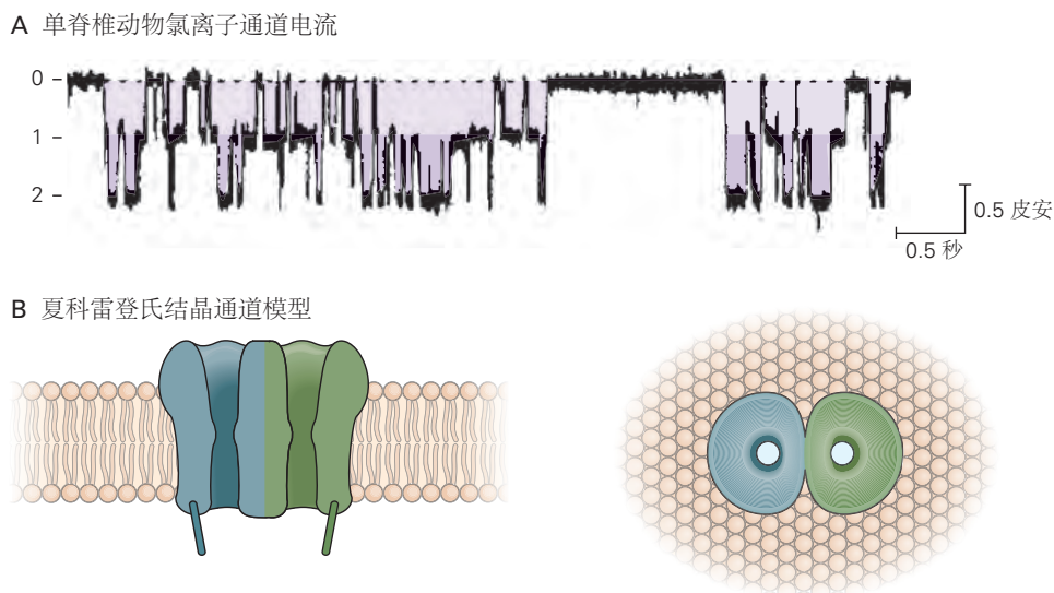
图 8.3.8: \text{Cl}^- 通道和转运蛋白的脊椎动物夏科雷登氏结晶家族是具有 2 个相同孔的双桶通道。A. 通过单个脊椎动物 \text{Cl}^- 通道的电流记录显示 3 个级别的电流：2 个孔都关闭 (0)、1 个孔打开 (1)，2 个孔都打开 (2)。B. 从侧面 (左) 显示通道并从细胞外向上看膜 (右)。每个亚基都包含自己的离子传输通路和门。此外，二聚体有 1 个由 2 个亚基共享的门 (未显示)。
