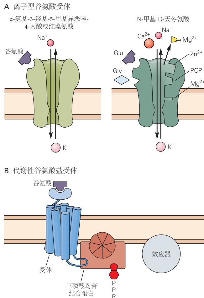
图 13.3.1: 不同类别的谷氨酸受体调节脊髓和大脑神经元中的兴奋性突触动作。A. 离子型谷氨酸受体直接门控可渗透阳离子的离子通道。AMPA 和红藻氨酸类型分别结合谷氨酸激动剂 AMPA 或红藻氨酸盐；这些受体包含一个可渗透 Na + 和 K + 的通道。NMDA 受体结合谷氨酸激动剂 NMDA；它包含 1 个可渗透 Ca 2+ 、K + 和 Na + 的通道。它具有谷氨酸、甘氨酸、Zn 2+ 、苯环利定、佐环平/地卓西平和 Mg 2+ 的结合位点，其中每一种都以不同方式调节通道的功能。B. 谷氨酸与代谢型谷氨酸受体的结合通过激活三磷酸鸟苷结合蛋白间接门控离子通道，三磷酸鸟苷结合蛋白又与效应分子相互作用，从而改变代谢和离子通道活性（第 11 章）。
