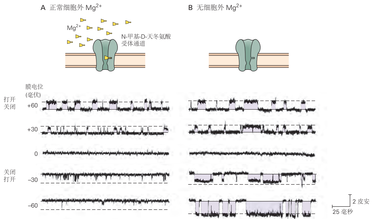
图 13.3.6: 除了谷氨酸之外，单个 NMDA 受体通道的打开还取决于膜电位。这些膜片钳记录来自单个 NMDA 受体通道（来自培养的大鼠海马细胞）。向下偏转表示内向（负）电流脉冲；向上偏转表示向外（正）电流。A. 当 Mg^{2+} 以正常浓度存在于细胞外溶液（1.2 毫摩尔）时，该通道在静息电位（-60 毫伏）处大部分被阻断。在负膜电位下，由于 Mg^{2+} 阻断，在通道打开时只能看到短暂、闪烁的内向电流。对 0 毫伏反转电位（至 +30 毫伏或 +60 毫伏）正电压的大量去极化解除了 Mg^{2+} 阻滞，允许更持久的外向电流脉冲通过通道。B. 当 Mg^{2+} 从细胞外溶液中去掉时，通道的打开和关闭不依赖于电压。如图 13.3.7B 所示，通道在 -60 毫伏的静息电位下打开，突触电流在接近 0 毫伏时反转，就像总突触电流一样。
