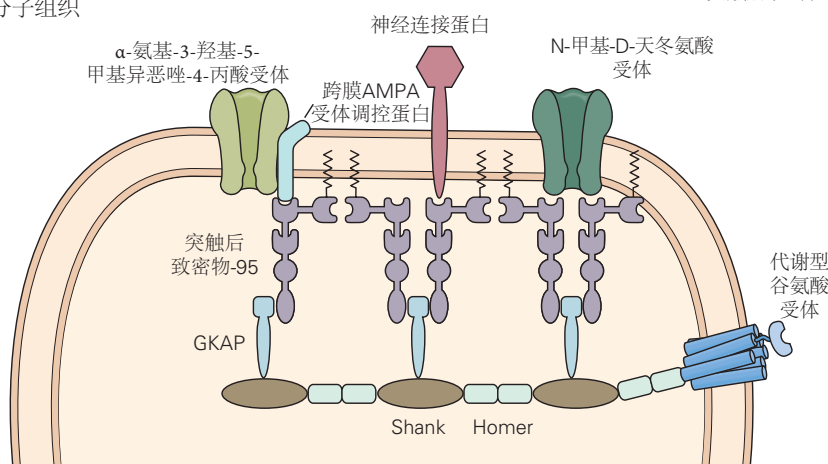
图 13.3.5: 突触后细胞膜在兴奋性突触处组织成大分子复合物。含有 PDZ 结构域的蛋白质有助于组织 AMPA 和 NMDA 谷氨酸受体在突触后密度的分布 [74] 。A. 生化纯化的突触后密度的电子显微镜图像，显示蛋白质网络的组织。膜脂双层不再存在。左图：通常是细胞外部的突触后密度视图。该图像由各种受体和膜蛋白的细胞外结构域组成。右图：从通常是膜的细胞质侧的突触后密度视图。白点显示免疫标记的鸟苷酸激酶锚定蛋白，这是突触后密度的重要组成部分。B. NMDA 受体、AMPA 受体和突触后致密物-95（一种突出的突触后密度蛋白）在突触处的分布。C. 受体网络及其在突触后密度中的相互作用蛋白。突触后致密物-95 在其氨基末端包含 3 个 PDZ 结构域，在其羧基末端包含 2 个其他蛋白质相互作用基序，1 个 SH3 域和一个鸟苷酸激酶结构域。突触后致密物-95 的某些 PDZ 结构域与 NMDA 受体的 GluN2 亚基的羧基末端结合。突触后致密物-95 不直接与 AMPA 受体相互作用，而是与膜蛋白跨膜 \alpha -氨基-3-羟基-5-甲基-4-异恶唑丙酸受体调控蛋白家族的羧基末端结合，后者作为辅助亚基与 AMPA 受体相互作用。突触后致密物-95 还通过与鸟苷酸激酶相关蛋白结合作为各种细胞质蛋白的支架，鸟苷酸激酶相关蛋白与突触蛋白 Shank 相互作用，突触蛋白 Shank 是一种结合成网状结构的大蛋白，连接突触后密度的各种成分。突触后致密物-95 还与神经连接蛋白的细胞质区域相互作用。代谢型谷氨酸受体位于突触的外围，在那里它与突触后密度蛋白 Homer 相互作用，后者又与突触蛋白 Shank（多结构域的骨架蛋白）结合。
