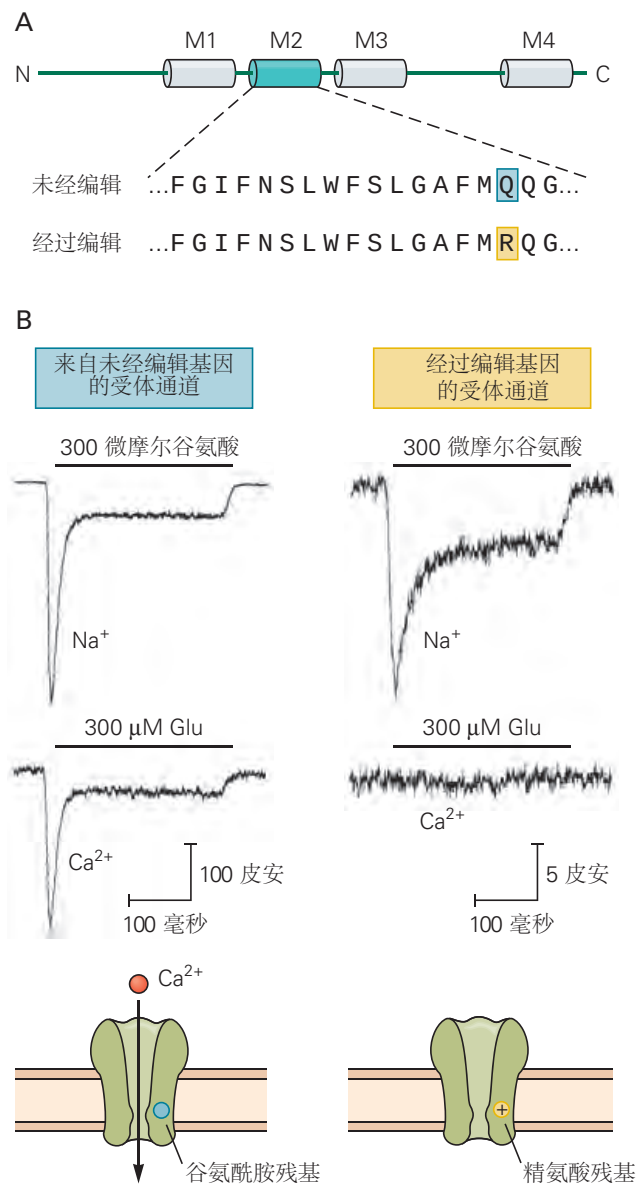
图 13.3.4: AMPA 受体通道 \text{Ca}^{2+} 渗透性的决定因素。A. 核糖核酸编辑前后 GluA2 基因编码的 AMPA 受体通道 M2 区氨基酸序列比较。未经编辑的转录本编码极性残基谷氨酰胺 (Q, 单字母氨基酸符号), 而编辑的转录本编码带正电的残基精氨酸 (R)。在成人中, GluA2 蛋白几乎完全以经过编辑的形式存在。B. 未经编辑的转录物表达的 AMPA 受体通道传导 \text{Ca}^{2+} (左迹线), 而经编辑的转录物表达的 AMPA 受体通道则不会 (右迹线)。迹线显示谷氨酸以细胞外 \text{Na}^+ (顶部) 或 \text{Ca}^{2+} (底部) 作为主要渗透阳离子引起的电流 [73] 。
