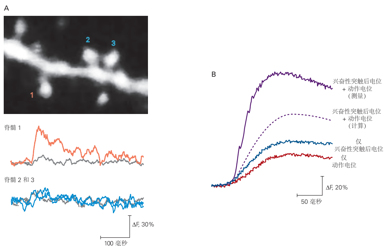
图 13.6.6: 树突棘通过 NMDA 受体分隔 \text{Ca}^{2+} 流入。A. 这张充满钙敏感染料的海马体阿蒙角 1 锥体神经元的荧光图像显示了具有多个棘的树突轴轮廓。当染料结合 \text{Ca}^{2+} 时，其荧光强度会增加。在突触前轴突的细胞外刺激后，这些痕迹绘制了一段时间内的荧光强度。脊柱 1 显示响应突触刺激（红色迹线）的荧光（ \Delta F ）大量快速增加，反映了通过 NMDA 受体的 \text{Ca}^{2+} 流入。相反，相邻树突轴（灰色迹线）的荧光强度几乎没有变化，表明 \text{Ca}^{2+} 积累仅限于脊柱头部。脊柱 2 和 3 显示出对突触刺激的荧光几乎没有增加，因为它们的突触前轴突没有被激活 [80] 。B. 当突触刺激与突触后动作电位配对时，脊柱中的钙积累最多。同时诱发兴奋性突触后电位和反向传播动作电位时生成的 \text{Ca}^{2+} 信号大于单独诱发兴奋性突触后电位或反向传播动作电位时单个 \text{Ca}^{2+} 信号的预期总和 [81] 。
