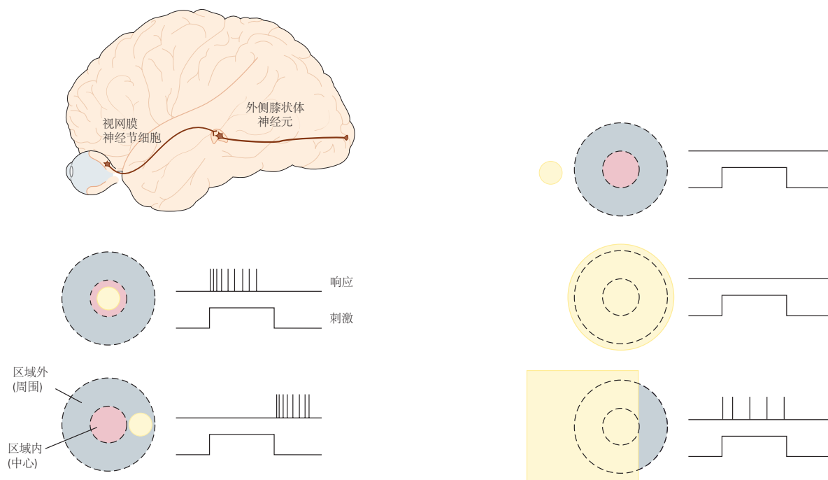
图 21.4.2: 视觉通路早期中继神经元的感受野。具有相互对立的中心和周围的圆形对称感受野是丘脑外侧膝状体核中视网膜神经节细胞和神经元的特征。中心可以响应光点（黄色）的打开或关闭，具体取决于感受野分别属于“在中心”还是“偏离中心”类。环绕具有相反的反应。在环绕之外，对光没有响应，从而定义了感受野边界。当光线同时覆盖中心和周围时，响应较弱，因此这些神经元对视野中的对比度（明暗边界）做出最佳响应。
