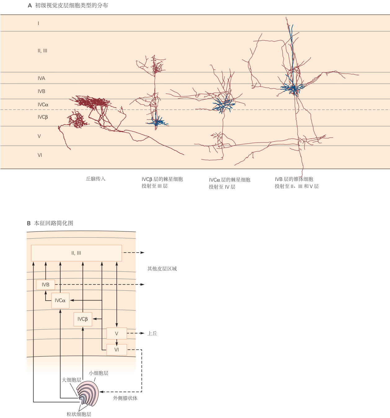
图 21.6.1: 初级视觉皮层的内在回路。A. 不同皮层中负责皮层回路兴奋性连接的神经元示例。第四层是来自丘脑外侧膝状体核的主要输入层。来自小细胞层的纤维终止于 IVC \beta 层，而大细胞纤维终止于 IVC \alpha 层。内在皮层兴奋性连接由多棘星形细胞和锥体细胞介导。多种 \gamma -氨基丁酸能平滑星形细胞（未显示）负责抑制连接。树突分枝是蓝色的，轴突分枝是棕色的 [188] 。B. 初级视觉皮层内的兴奋性连接图。从视觉皮层的每一层发送到皮层其他区域的输出。
