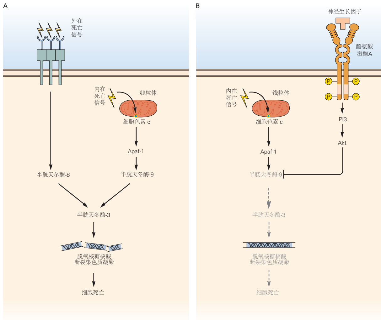
图 46.8.7: 神经营养因子抑制半胱天冬酶活化和细胞死亡 [422] 。A. 2 种类型的通路触发细胞死亡：表面膜死亡受体的外在激活和线粒体通路的内在激活。这 2 种通路都会导致 半胱天冬酶-8 和 半胱天冬酶-9 等 半胱天冬酶的激活，从而启动蛋白水解切割级联响应，该级联响应会聚在 半胱天冬酶-3 激活水平。半胱天冬酶前体的切割去除半胱天冬酶前结构域并产生蛋白水解活性酶构象。外在通路涉及配体激活死亡受体，例如肿瘤坏死因子受体 1 或 Fas/CD95。内在通路涉及应激诱导的信号，例如脱氧核糖核酸损伤，这些信号启动线粒体膜间隙释放细胞色素 c。细胞色素 c 与凋亡蛋白酶激活因子 1 结合并募集和激活半胱天冬酶-9。B. 神经营养蛋白与酪氨酸激酶受体的结合会募集磷酸肌醇 3-激酶通路和蛋白激酶 B，并通过抑制 半胱天冬酶-9 来抑制细胞死亡通路。该通路在神经元发育过程中被神经营养因子抑制，这解释了为什么这些因子的消除会导致细胞凋亡。
