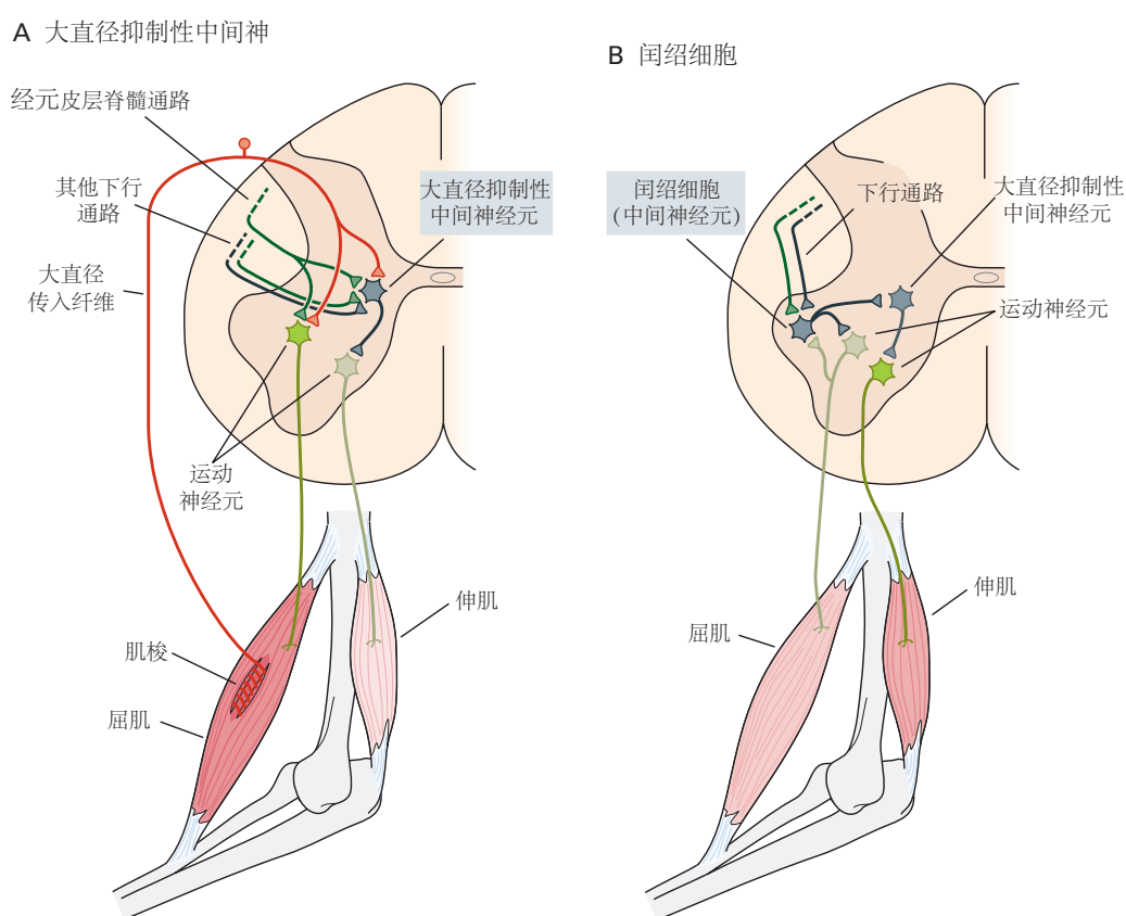
图 32.3.3: 抑制性脊髓中间神经元协调反射动作。 A. 大直径抑制性中间神经元通过与运动神经元的不同接触调节牵张反射回路中拮抗肌的收缩。此外，中间神经元接收来自皮层脊髓和其他下行通路的兴奋性和抑制性输入。这些脊髓上信号的平衡变化允许中间神经元协调关节处拮抗肌的共同收缩。 B. 闰绍细胞对运动神经元产生周期性抑制。这些中间神经元被来自运动神经元的侧支兴奋并抑制这些相同的运动神经元。这种负反馈系统调节运动神经元的兴奋性并稳定放电率。闰绍细胞还向协同运动神经元（未显示）和与拮抗运动神经元形成突触的大直径抑制性中间神经元发送侧枝。因此，调节闰绍细胞兴奋性的下行输入调节了控制关节周围运动的所有运动神经元的兴奋性。
