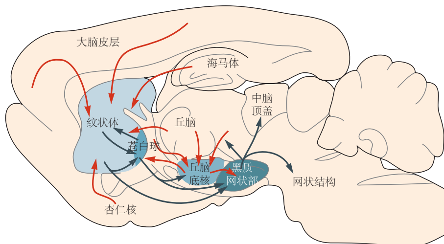
图 38.1.1: 哺乳动物基底神经节的主要输入连接、内部连接和输出连接。主 输入核 是纹状体、丘脑底核和黑质致密部（未显示）。它们直接接收来自大脑皮层、边缘结构（杏仁核和海马体）、丘脑的输入。主 输出核 是黑质网状部和内侧苍白球/脚内核（未显示）。外侧苍白球被归类为 内部核 ，因为它的大部分连接都与其他基底核相连。结构显示在啮齿动物大脑的矢状图上。红色和深灰色箭头分别表示 兴奋性连接 和 抑制性连接 。
