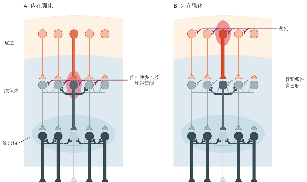
图 38.7.1: 2 个独立的强化机制可以在基底神经节的可重入并行循环结构中进行偏向选择（为清楚起见，省略了通过丘脑的回路返回连接）。 A. 内在强化（红色椭圆形）涉及皮层纹状体神经传递的选择性敏化（由不同通道中纹状体投射神经元的相对厚度表示）。最近活跃（选定）通道中的传输通过多巴胺和谷氨酸的联合相位性释放得到加强，该释放是由意外的生物学显著感觉事件（例如奖励）引起的。非活动通道缺乏突触多巴胺强化所需的资格迹。由此产生的选择可塑性将导致优先重新选择近期行为输出的强化版本，从而在行动和结果之间建立关联。 B. 最近的研究表明，与奖励（红色椭圆形）的关联可以加强向纹状体提供传入信号结构中的处理。就基底神经节的选择部分取决于输入到纹状体信号的相对强度（广泛接受的观点），与奖赏相关的传入信号调节实际上会选择偏向于奖励相关的输入。同样，图中投射的粗细表示激活的相对水平。
