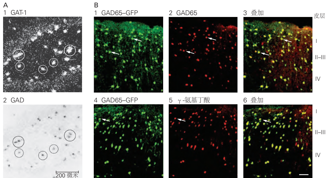
图 16.3.2: 可视化化学信使的技术。A. 大鼠海马体的光学显微镜切片。1. 使用编码γ-氨基丁酸转运蛋白 1 的信使核糖核酸的探针的原位杂交。用 \alpha -35S dATP 对探针进行末端标记，并通过覆盖的放射自显影照相乳剂中的银颗粒簇进行观察。2. 用与碱性磷酸酶连接的寡核苷酸探针对谷氨酸脱羧酶的信使核糖核酸进行原位杂交，谷氨酸脱羧酶是 γ-氨基丁酸的特异性生物合成酶。谷氨酸脱羧酶探针通过细胞质中有色碱性磷酸酶响应产物的积累而显现。表达γ-氨基丁酸转运蛋白-1 和谷氨酸脱羧酶转录物的神经元分别用银粒和磷酸酶响应标记，并用包含这 2 种标记的细胞体周围的圆圈表示。B. 来自谷氨酸脱羧酶 65-绿色荧光蛋白转基因小鼠的新皮层的图像，其中绿色荧光蛋白在谷氨酸脱羧酶 65 启动子的控制下表达。绿色荧光蛋白与谷氨酸脱羧酶 65 (1-3) 和γ-氨基丁酸 (4-6) (均通过间接免疫荧光检测) 共同定位于不同层的神经元中。大多数绿色荧光蛋白阳性神经元对谷氨酸脱羧酶 65 和γ-氨基丁酸呈免疫阳性 (箭头显示所选实例)。比例尺为 100 微米。
