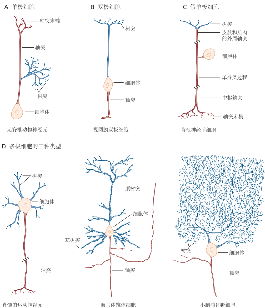
图 3.1.3: 根据源自细胞体的过程的数量，神经元分为单极、双极或多极。 A. 单极细胞有一个从细胞体发出的单一突起。不同的部分作为接受表面或释放末梢。单极细胞是无脊椎动物神经系统的特征。 B. 双极细胞有 2 种功能特化的突起。树突接收电信号，轴突将信号传递给其他细胞。 C. 伪单极细胞是双极细胞的变体，负责将体感信息传递到脊髓。在发育过程中，胚胎期双极细胞原有的 2 个突起融合，形成一个从细胞主体出发的单一过程，该过程具有 2 个功能不同的部分。2 个部分都起轴突的作用；一个延伸到外周皮肤或肌肉，另一个延伸到中枢脊髓 [19] 。 D. 多极细胞具有单个轴突和许多树突。它们是哺乳动物神经系统中最常见的神经元类型。以下 3 个例子说明了这些细胞的巨大多样性。脊髓运动神经元支配骨骼肌纤维。锥体细胞具有大致呈三角形的细胞体；树突从顶点（顶端树突）和基部（基底树突）出现。锥体细胞存在于海马体和整个大脑皮层中。小脑的浦肯野细胞以其丰富且广泛分布的树突网络为特点，能容纳数量庞大的突触输入 [19] 。
