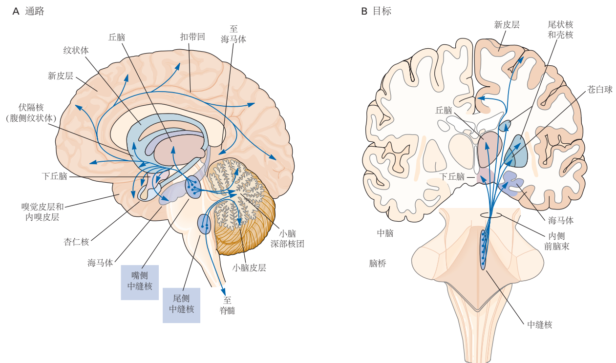
图 61.6.1: 大脑中的主要 5-羟色氨酸系统出现在脑干的中缝核中。5-羟色氨酸在一组称为中缝核的脑干核中合成。这些神经元投射到整个神经轴，范围从前脑到脊髓。5-羟色氨酸能投射是单胺能系统中最庞大和最分散的，单个 5-羟色氨酸能神经元支配数百个目标神经元 [21] 。A. 大脑的矢状面图显示了中缝核。在大脑中，这些细胞核形成了一个相当连续的细胞群集合，靠近脑干中线并沿其长度延伸。在这里的图中，它们以更明显的嘴侧和尾侧组显示。头侧中缝核投射到大量的前脑结构。B. 这张大脑的冠状视图说明了由 5-羟色氨酸能中缝核神经元支配的一些主要结构。
