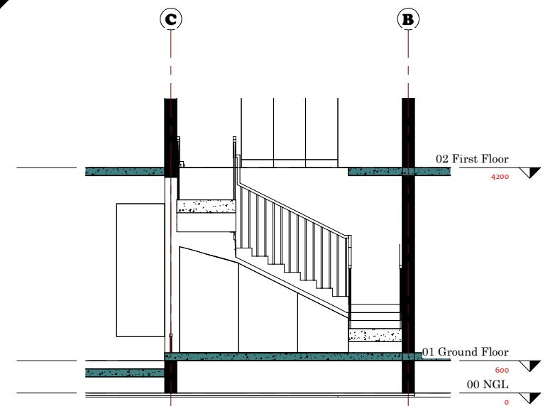
2 Section 3 1 : 50
