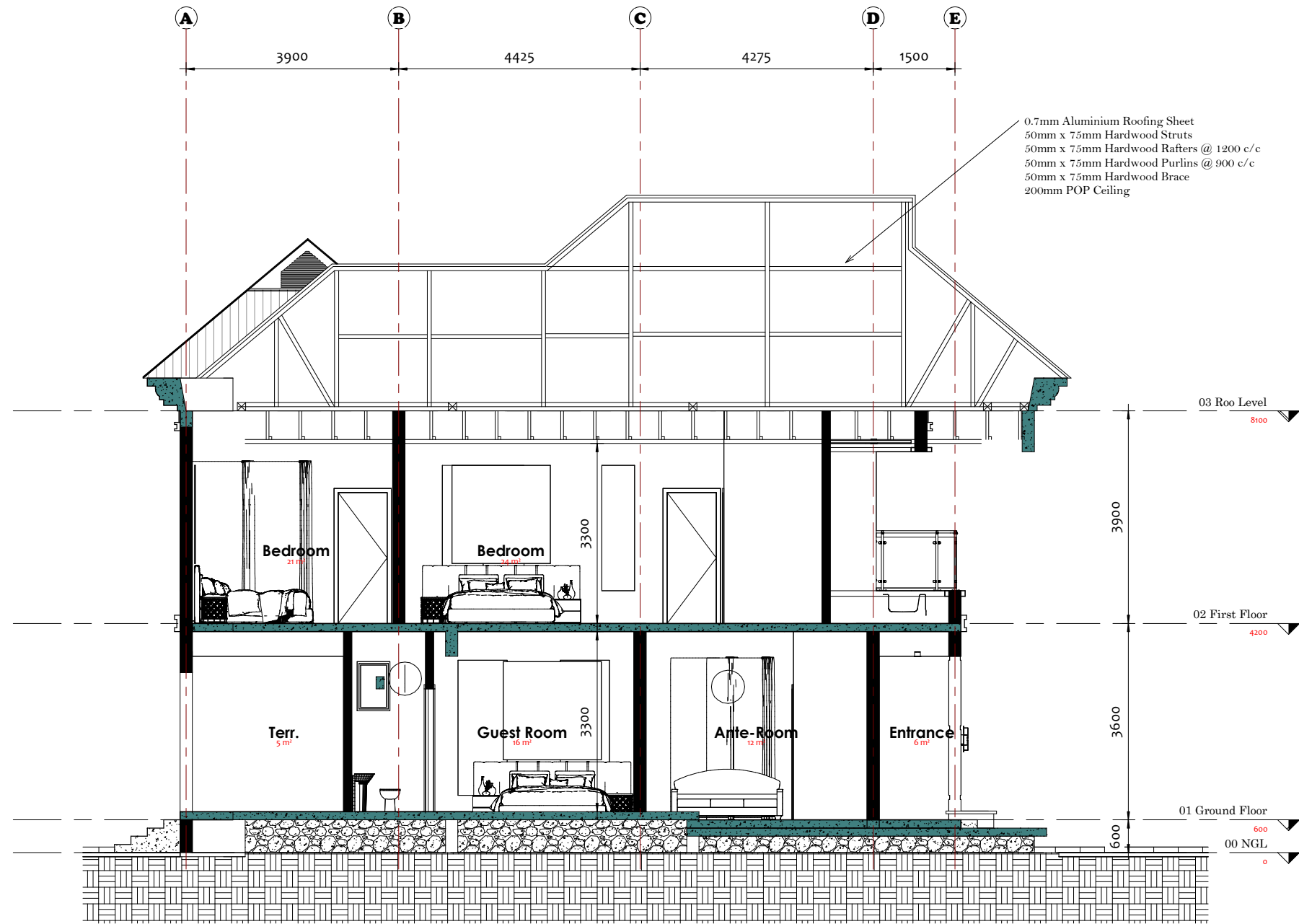
1 Section 2 1 : 50
