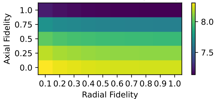
Max Skewness
