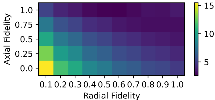
Max Skewness
