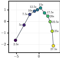
MOSS-Audio L18
