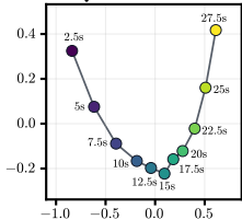
Qwen3-Omni L24
