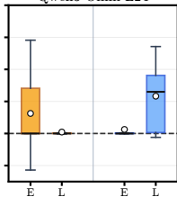
Qwen3-Omni L24
