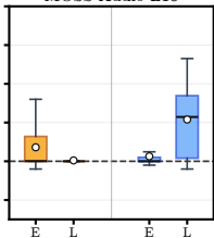
MOSS-Audio L18
