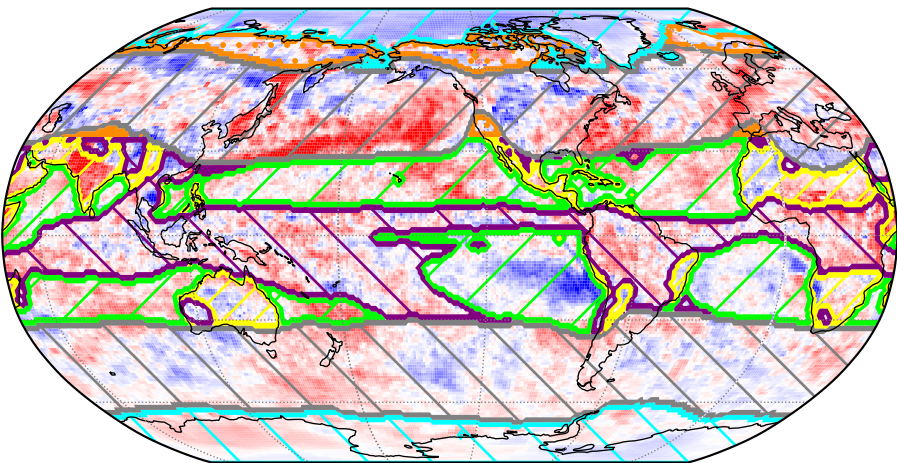
a) MAM = 0.46
