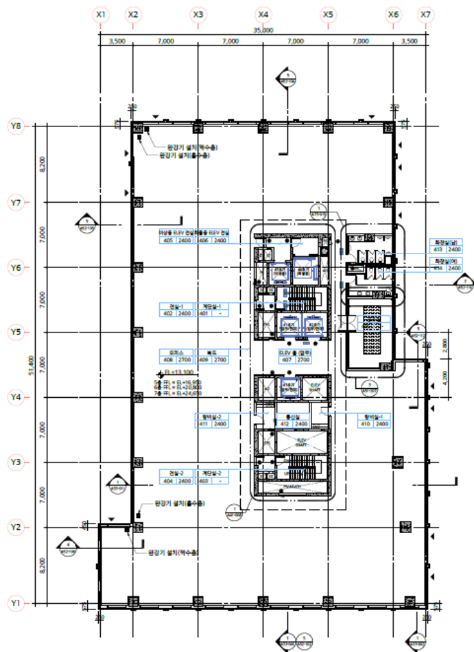
■ 평면도 (7층)
