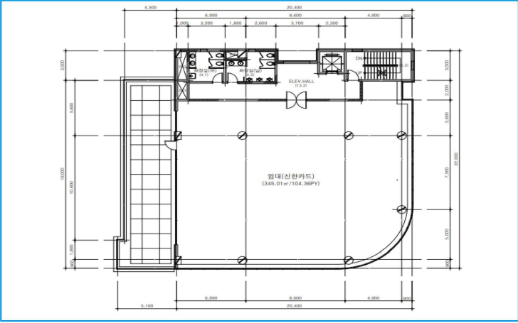
<기준층 평면도> (단위: 평,원)
