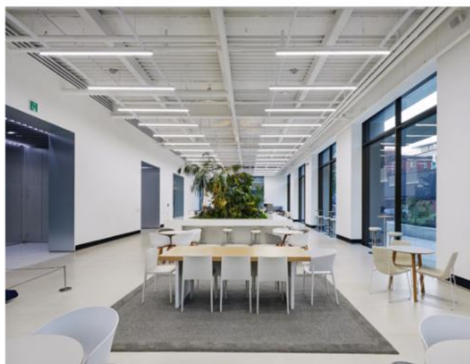
▲ 1F CAFÉ
