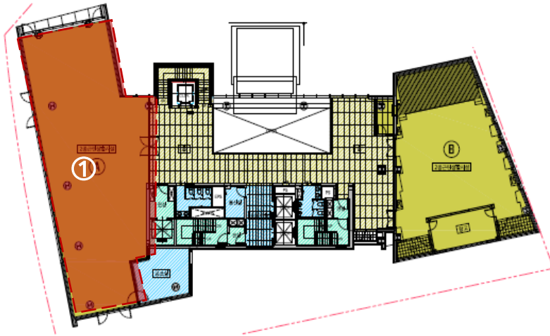
도면(5,6F)
