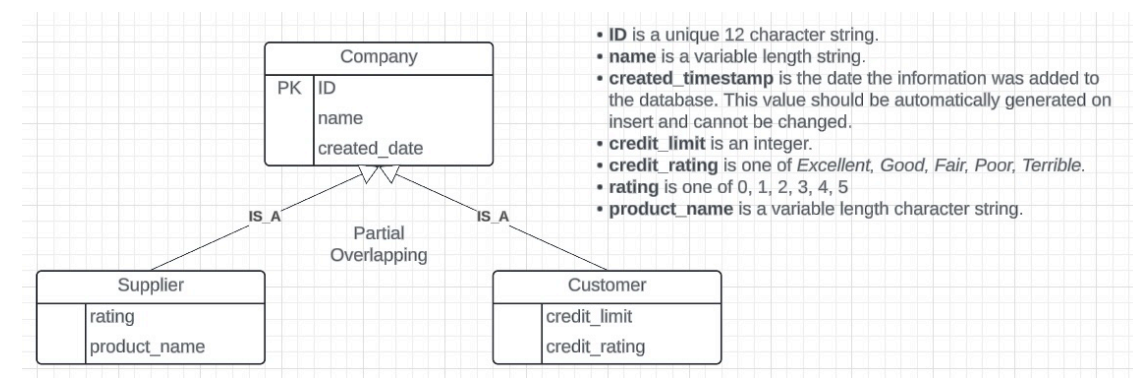
ER to SQL Data Model
