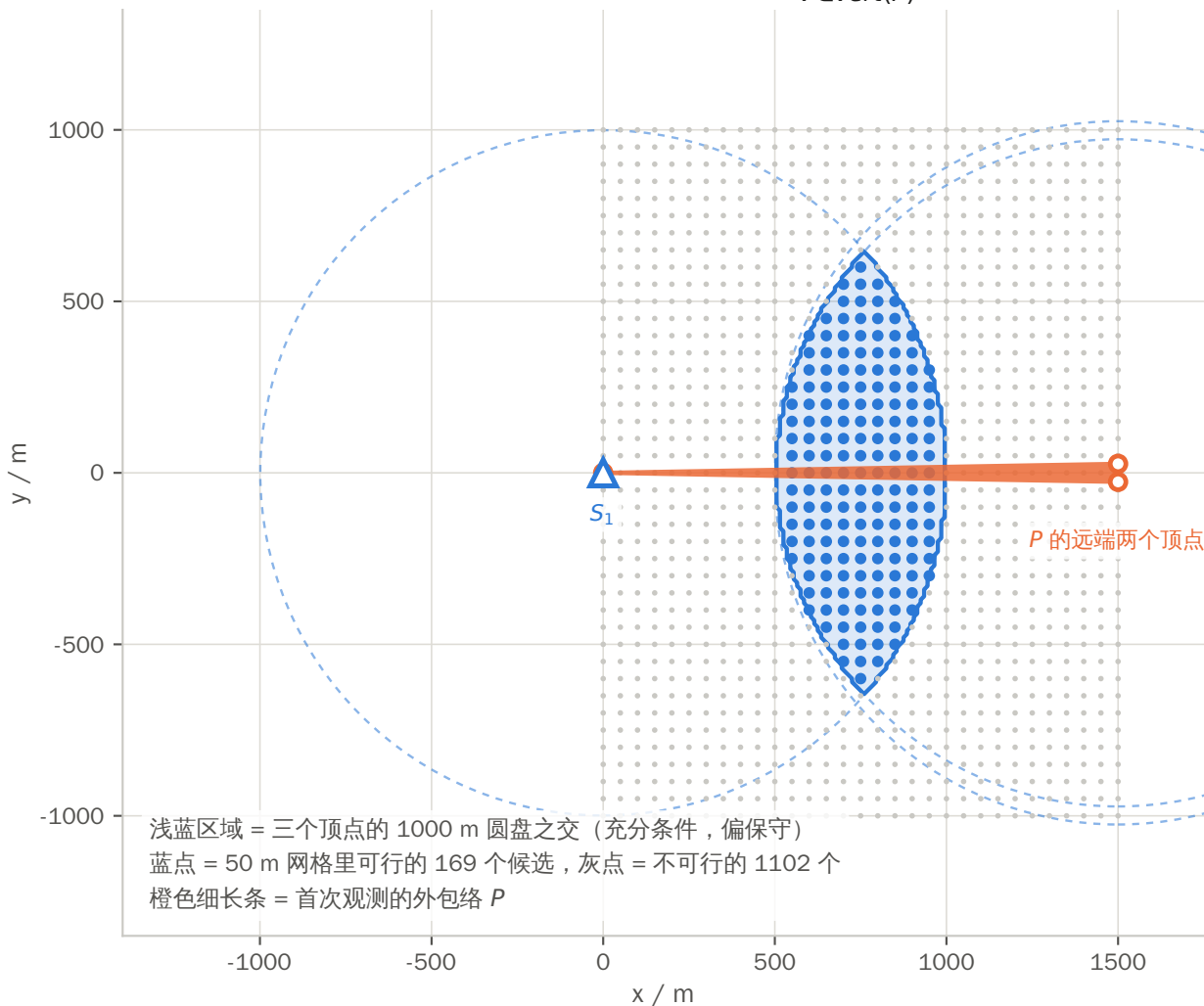
图 6 第二检测点的安全候选域 C_{safe} = \{S: \max_{V \in \text{vert}(P)} |S-V| \leq 1000 \text{ m}\}
