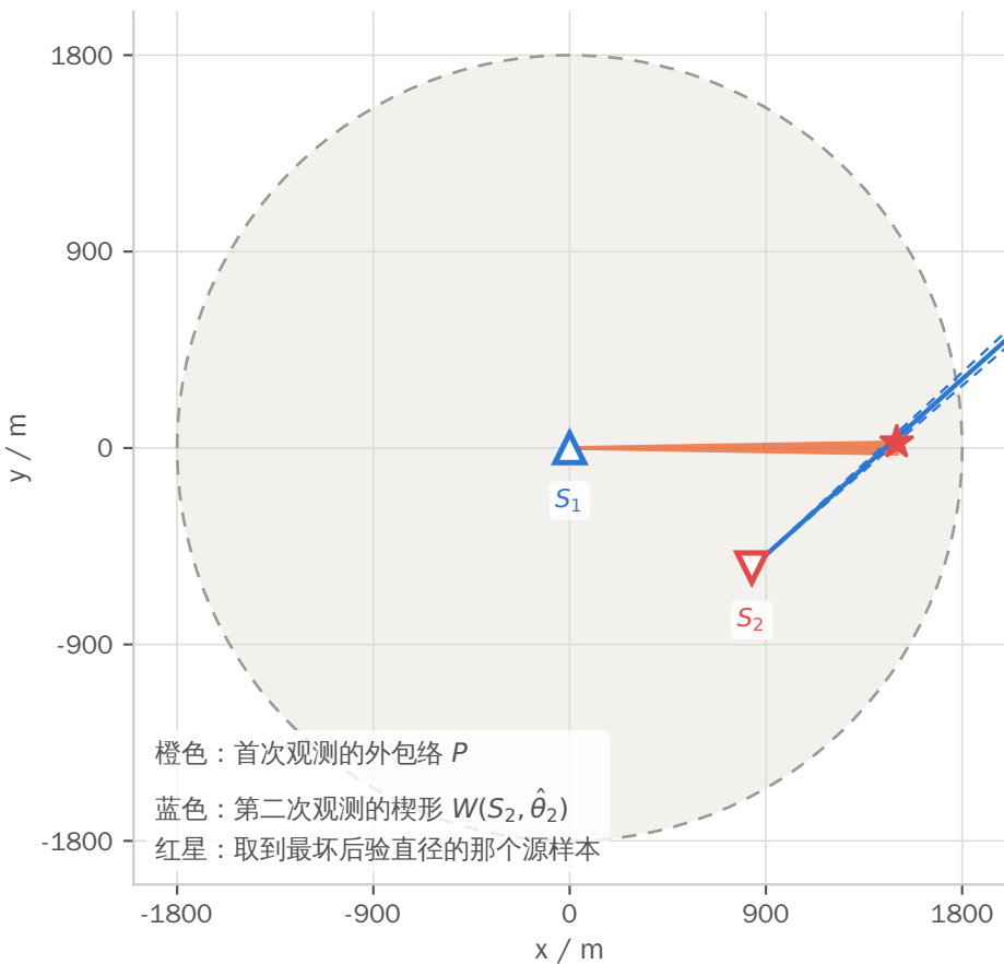
(a) 两条方位线的交会
