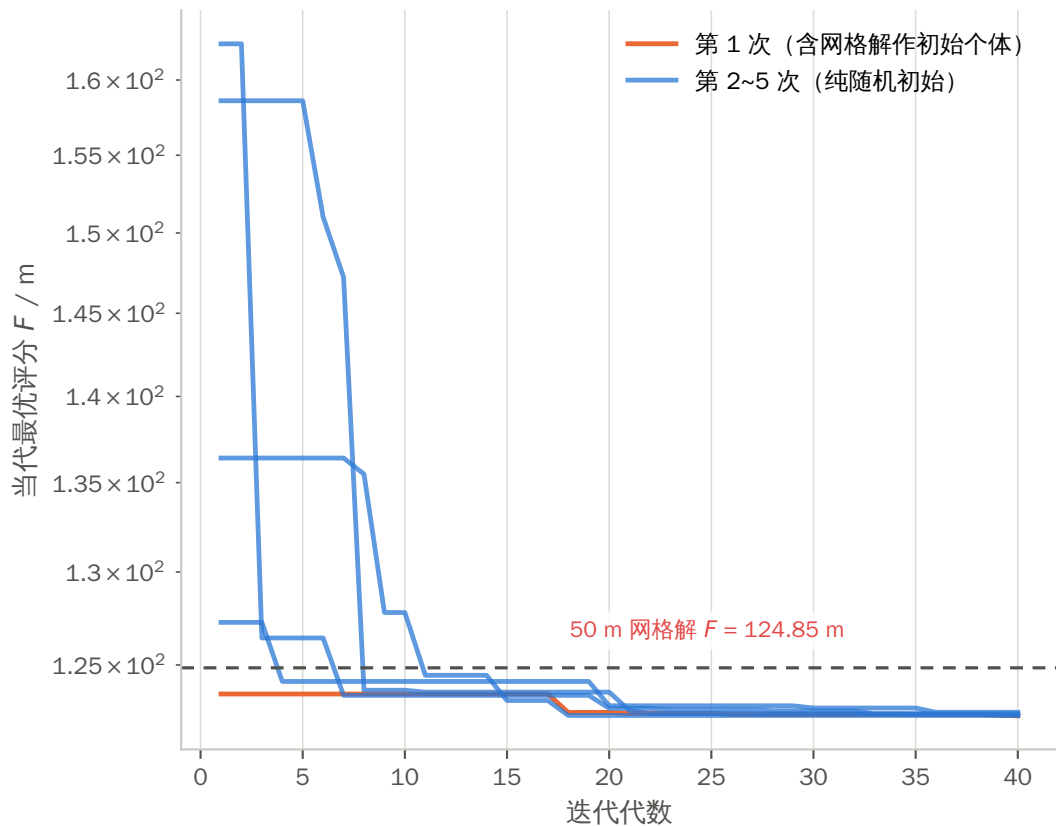
(a) 5 次独立运行的收敛曲线 (纵轴对数)
