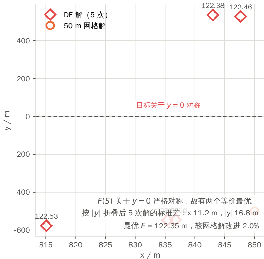
(b) 解落在两个镜像最优上
