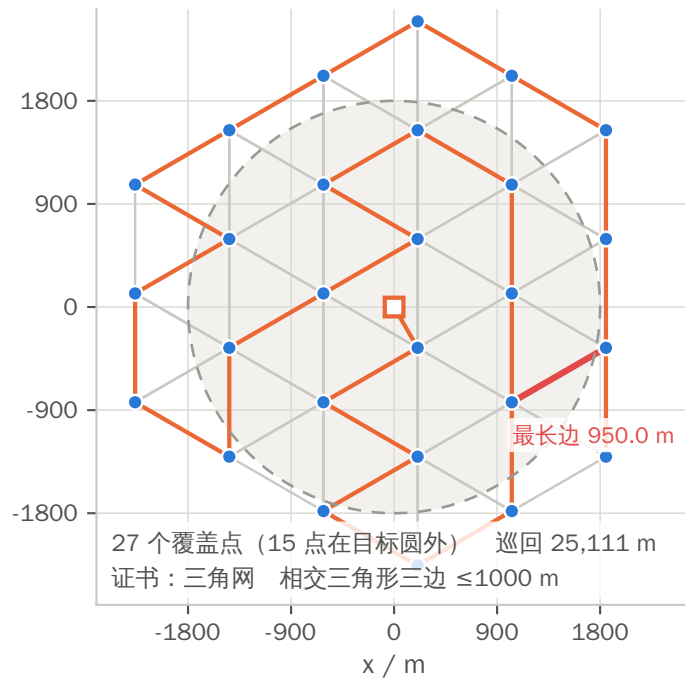
(b) 问题四·方案四 规则三角格 h=950 m
