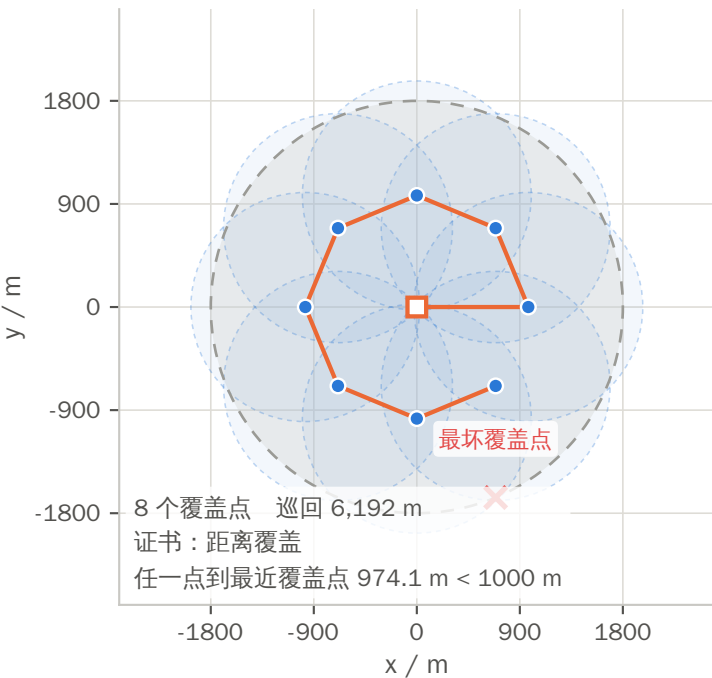
(a) 问题三·正八边形覆盖网
