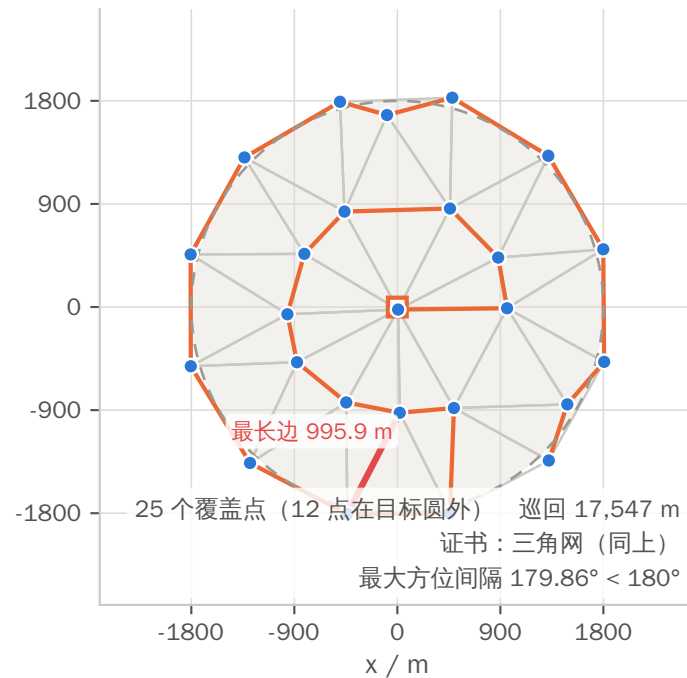
(c) 问题四·方案七 非规则三角网
