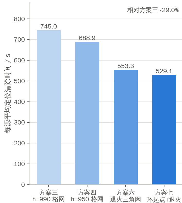
(c) 接进求解器后的实际时间 (问题四训练集)
