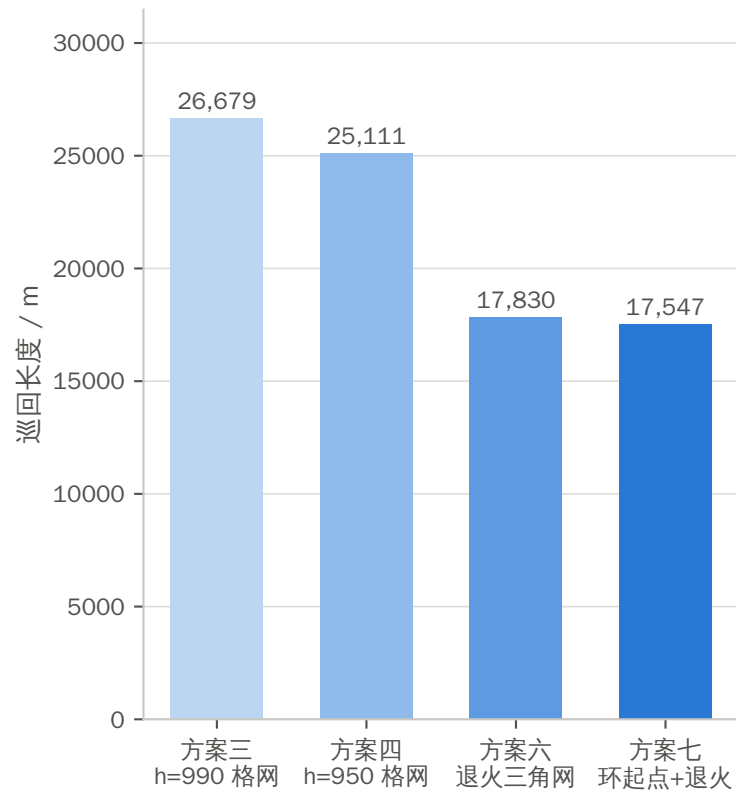
(a) 巡回长度：26.7 km → 17.5 km
