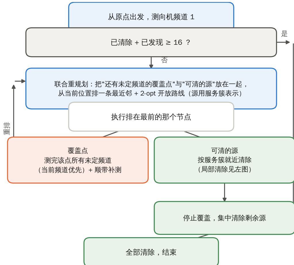
(b) 主循环 (方案七 = 方案六的调度 + 25 点覆盖网)
