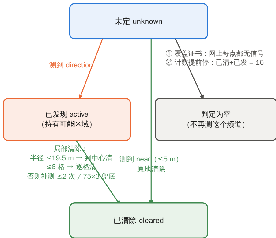
(a) 频道状态机 (20 个频道各自独立)
