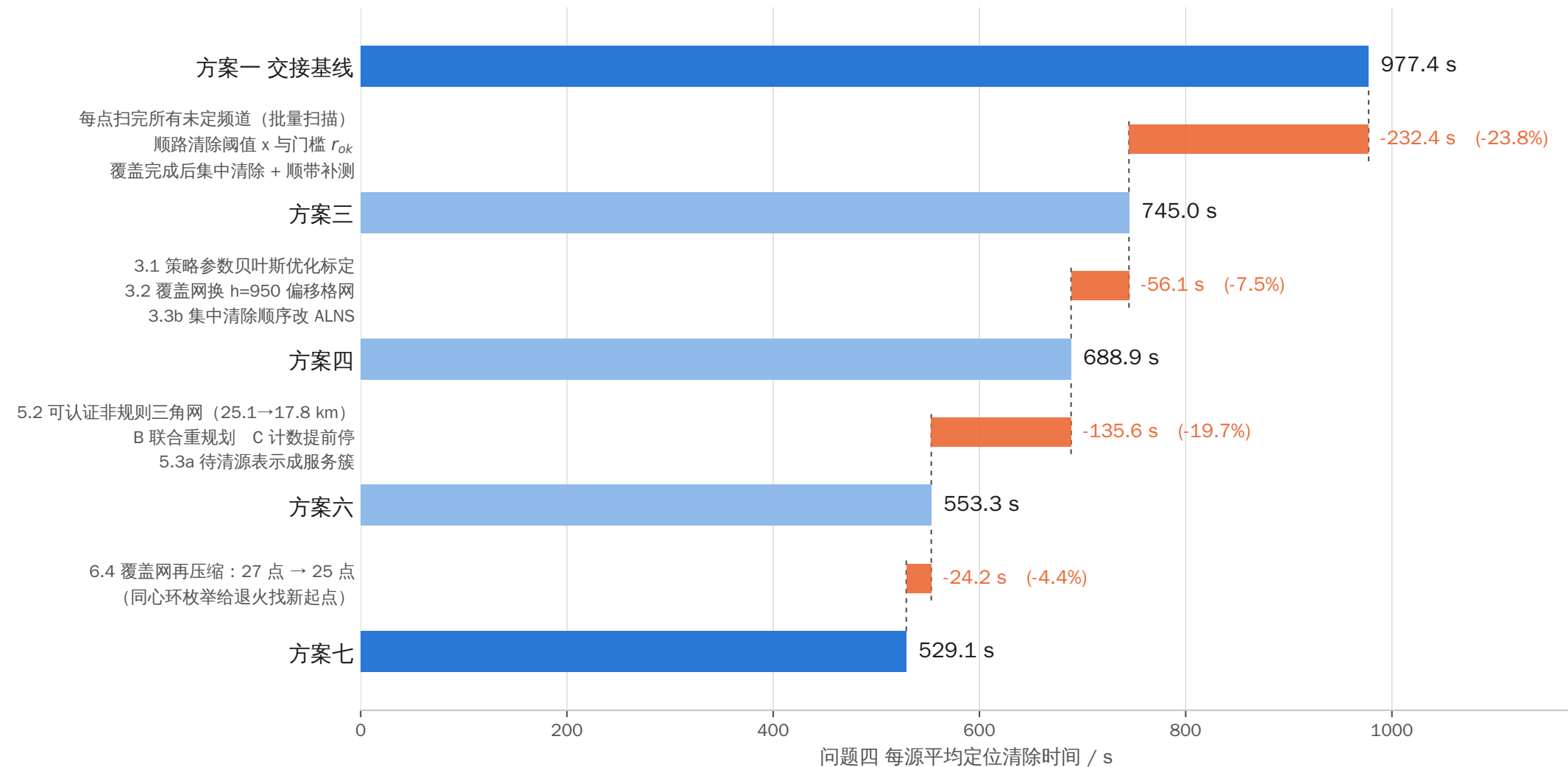
图 20 问题四的优化过程：977.4 s → 529.1 s (累计 -45.9%)
