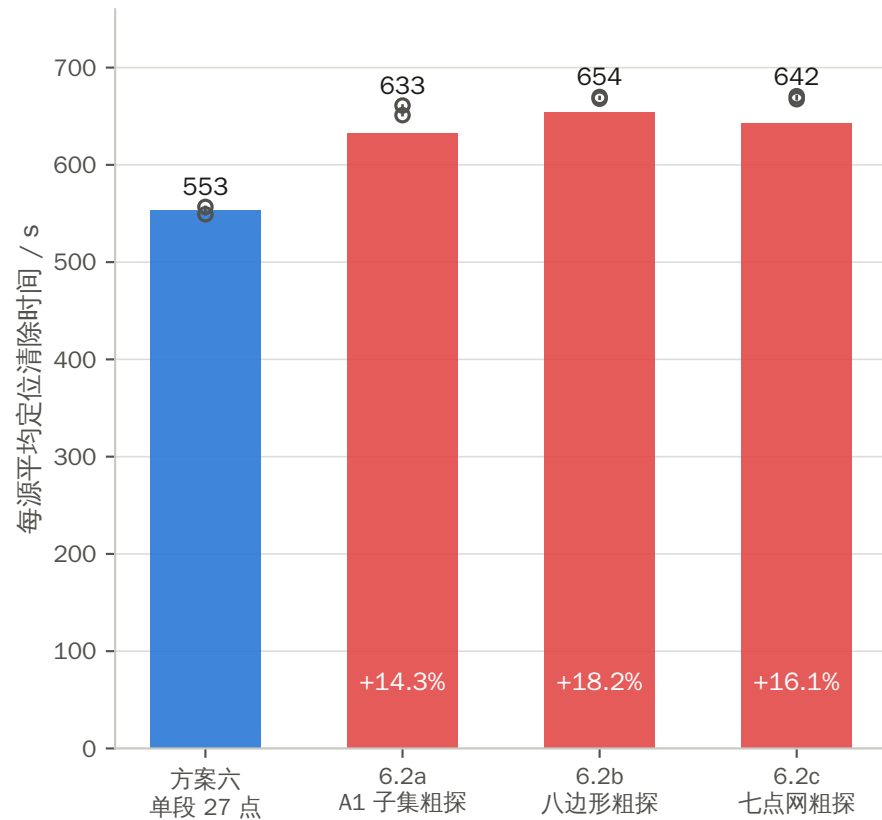
(b) 三种粗探集都更慢 (柱 = 训练集, 点 = 验证集)
